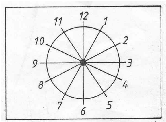
Сл.2: Подела данцета чауре на сегменте
