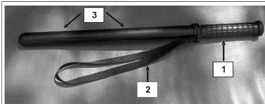
Основни делови службене палице су: Рукохват (1), најлонска трака (2) и тело палице (3)
